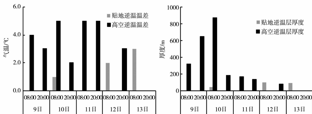
图5 榆中2013年3月9~13日逆温温差(左)与逆温层厚度(右)
